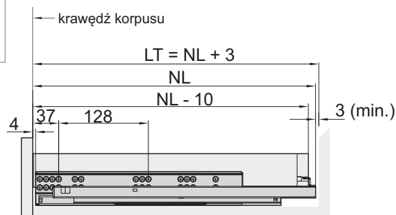
szuflada z frontem nakładanym
