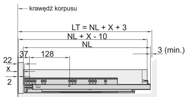
szuflada z frontem wpuszczanym
